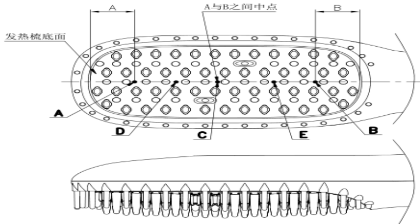
图6 热直发梳温度测量点置
