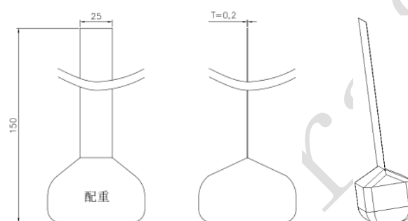
图8 测试纸带
