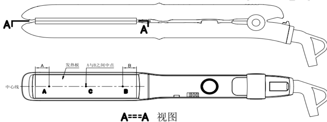
图4 直发器温度测量点位置
