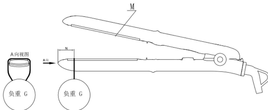
图9 铰轴吊磅
