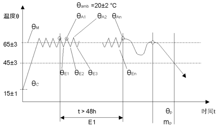
图 4 24h 固有能耗与热水输出率的测试程序示意
