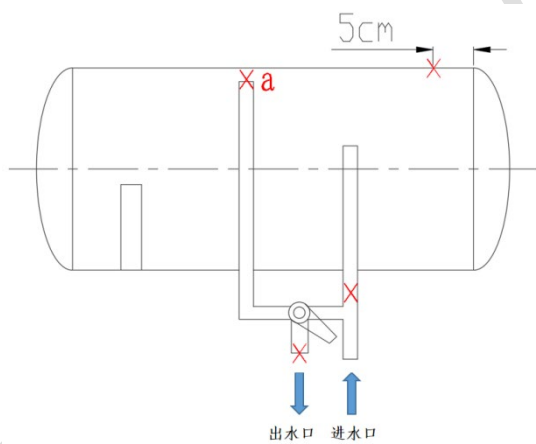
图 6(a) 卧式安装的热热水器的热电偶放置位置
